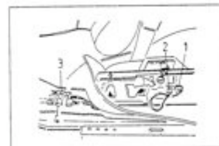
Bild 362 Anschlüsse Steuereinheit 1-4 Kabelbox
